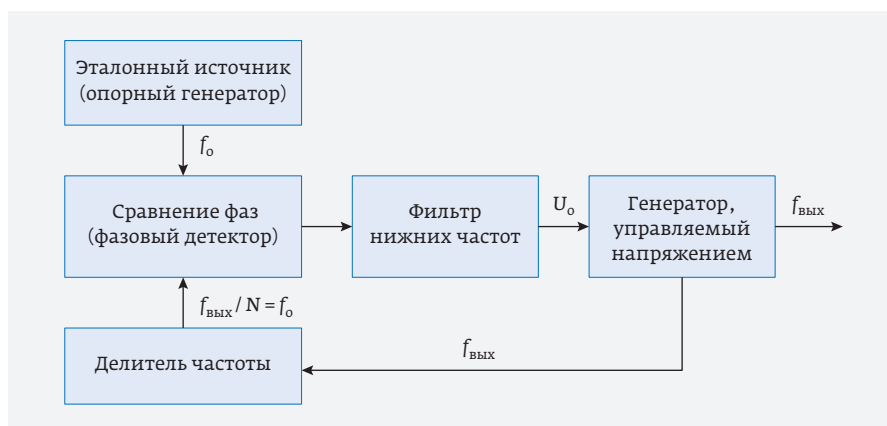
Рис. 38. Функциональная схема генератора с ФАПЧ с аналоговой системой формирования управляющего напряжения U_0 ГУН
