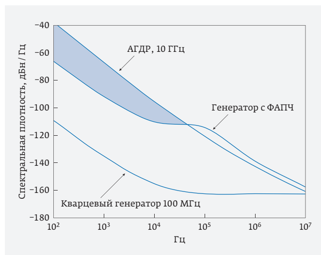
Рис. 39. Пример спектральной плотности фазовых шумов АГДР, генератора с ФАПЧ и кварцевого генератора
